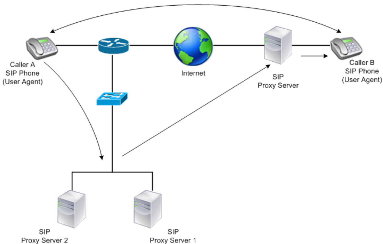
図 1: SIP ベースの通信システム
