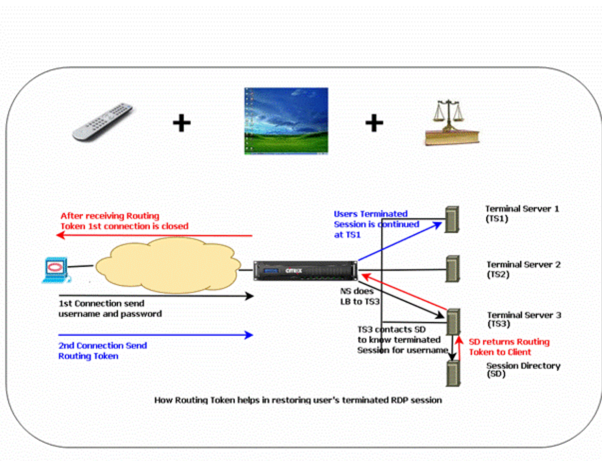
図 1: RDP のロードバランシングトポロジ
