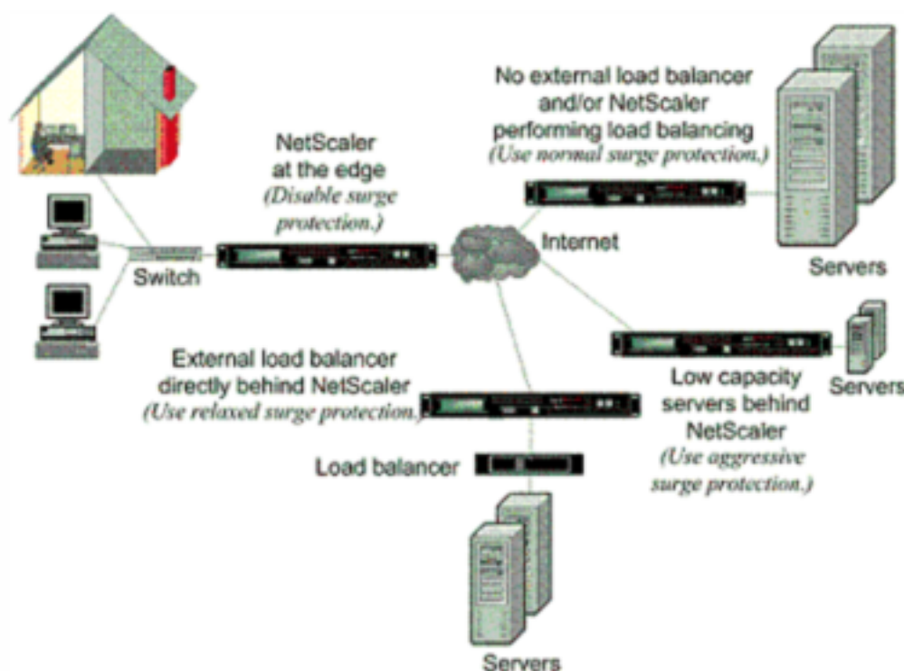
図 1: Citrix ADC サーージ保護の機能図
