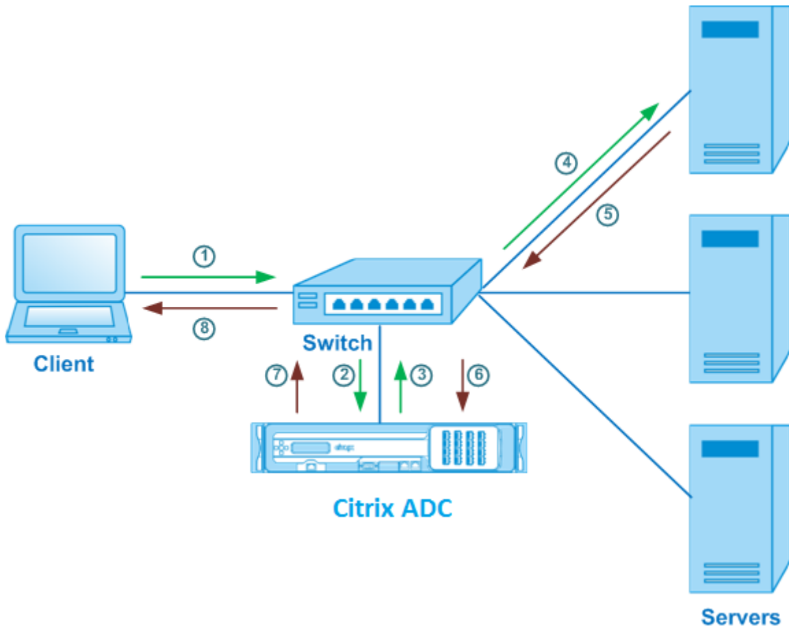
図 1: ワンアームモードでのロードバランシング
