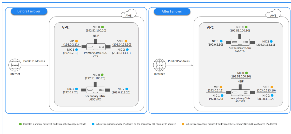
図 1: プライベート IP マイグレーションを使用した、AWS 上の Citrix ADC VPX HA ペア
