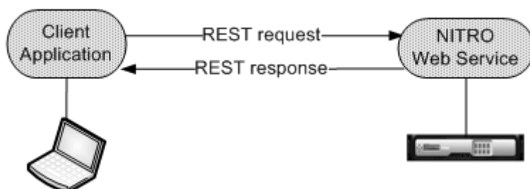
Abbildung 1. NITRO-Workflow
