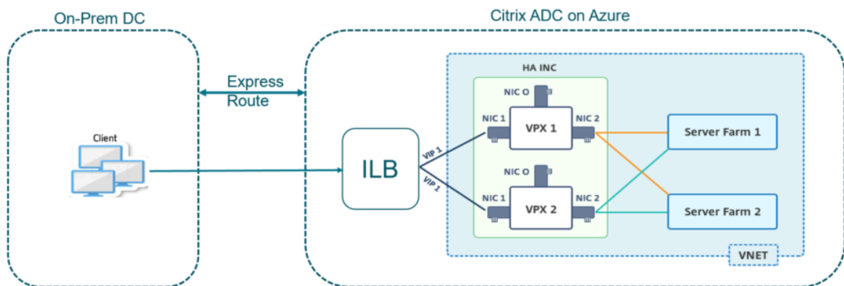
Abbildung 1: Citrix ADC HA-Paar für Clients in einem internen Netzwerk
