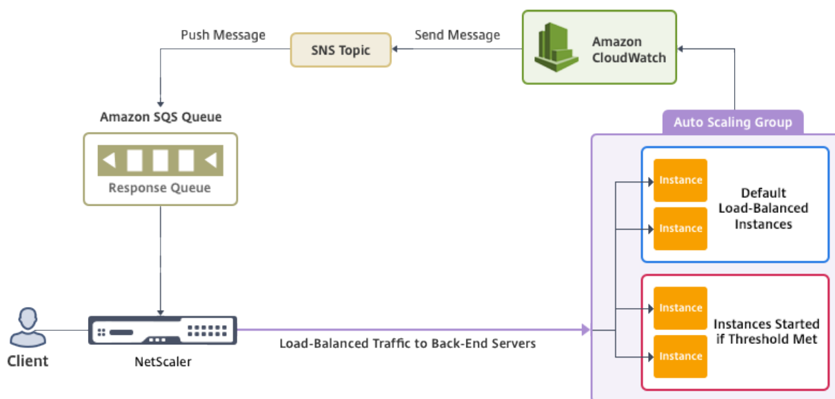
Diagramm: AWS Autoscaling Service mit einer Citrix ADC VPX Instanz
