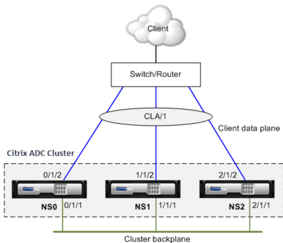
Abbildung 1. Cluster-Link-Aggregationstopologie
