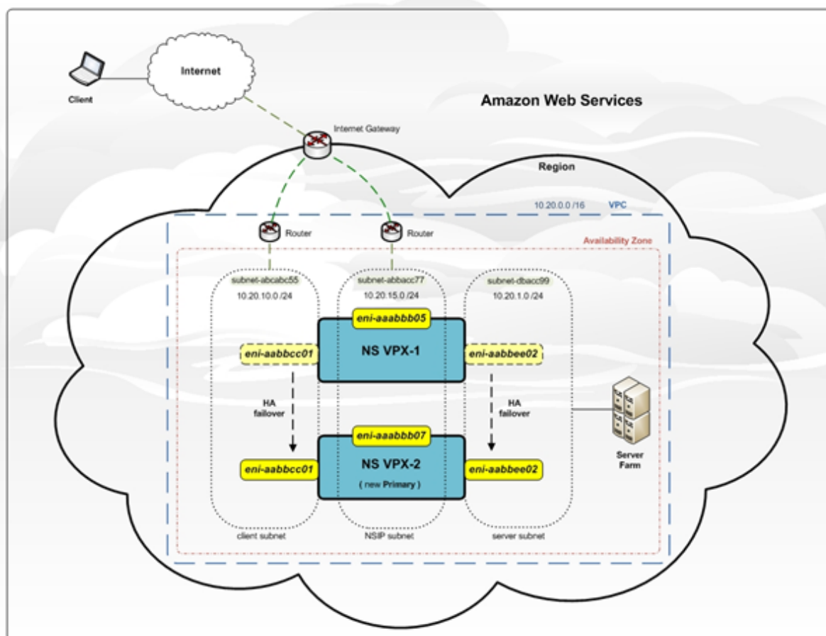
Abbildung 1. Ein Citrix ADC VPX HA-Paar in AWS mit ENI-Migration
