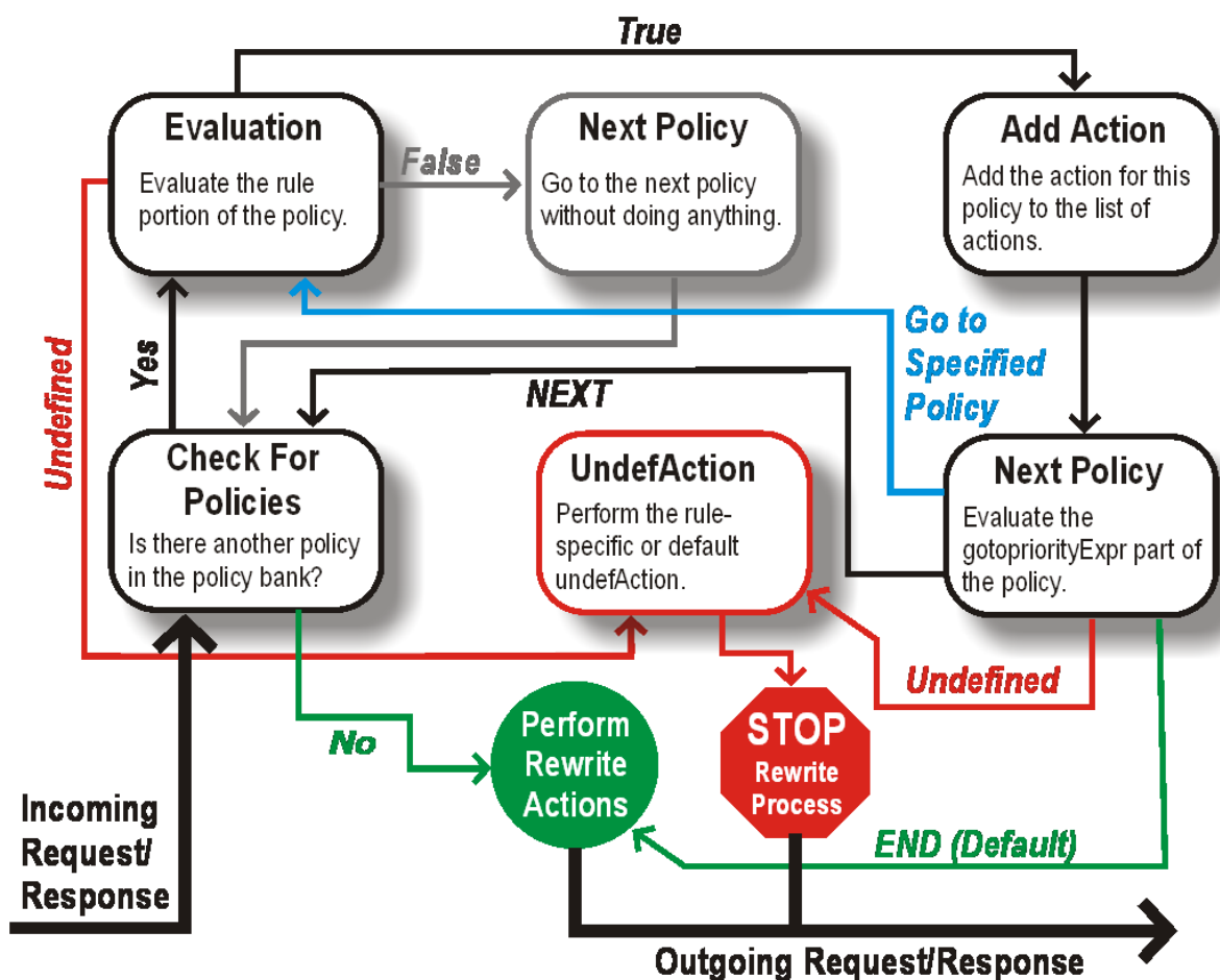
Abbildung 1. Der Rewrite-Prozess
