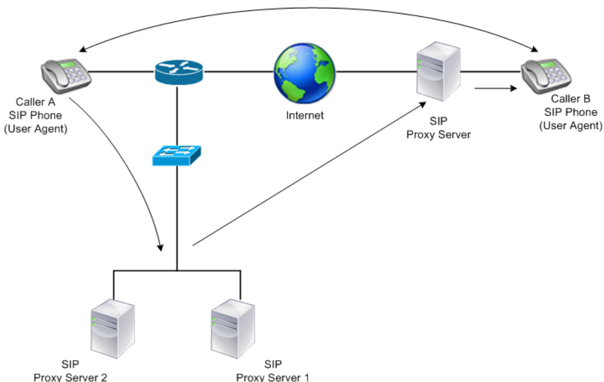
Abbildung 1. SIP-basiertes Kommunikationssystem
