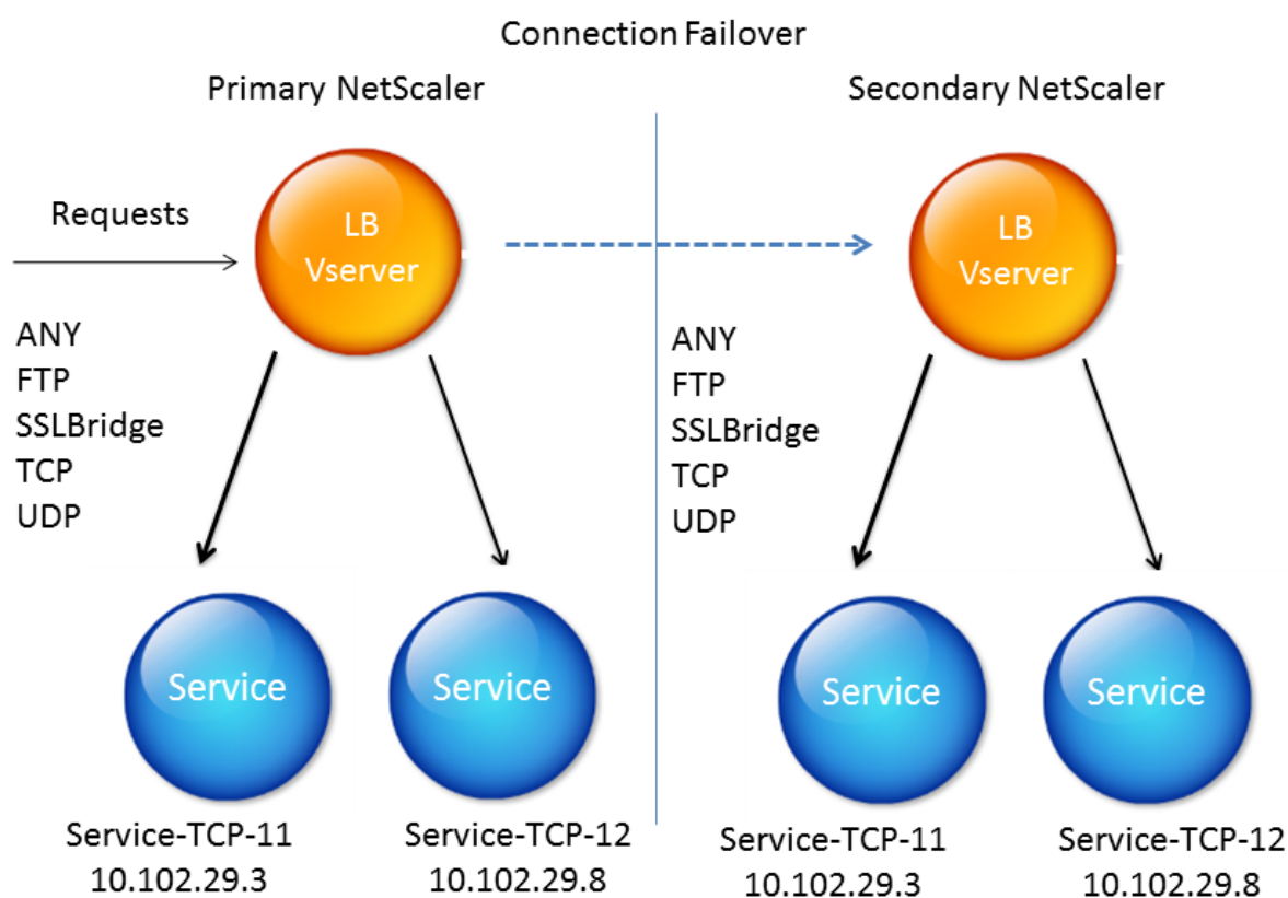
Abbildung 1. Verbindungs-Failover-Entitätsdiagramm
