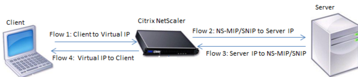
Abbildung 1. Citrix ADC-Flowsequenz
