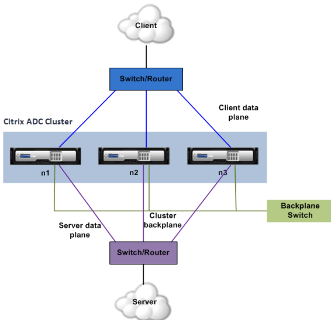
Abbildung 3. Clusterkommunikationsschnittstellen - L3-Cluster
