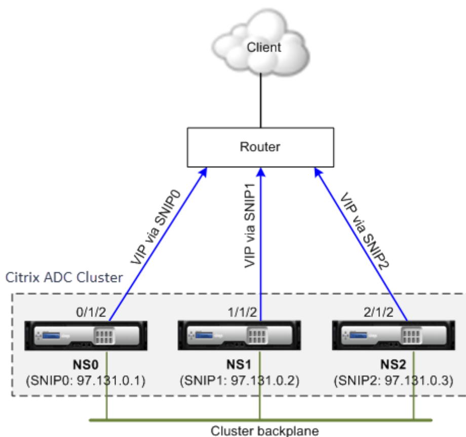
Abbildung 1. ECMP-Topologie
