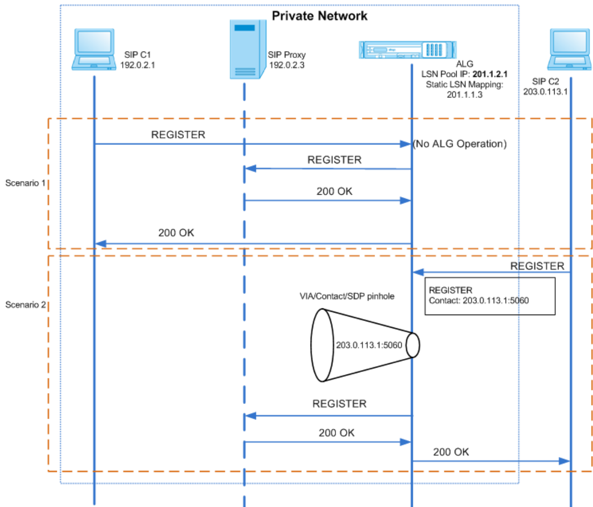
Abbildung 2. SIP-Eingehender Anruf
