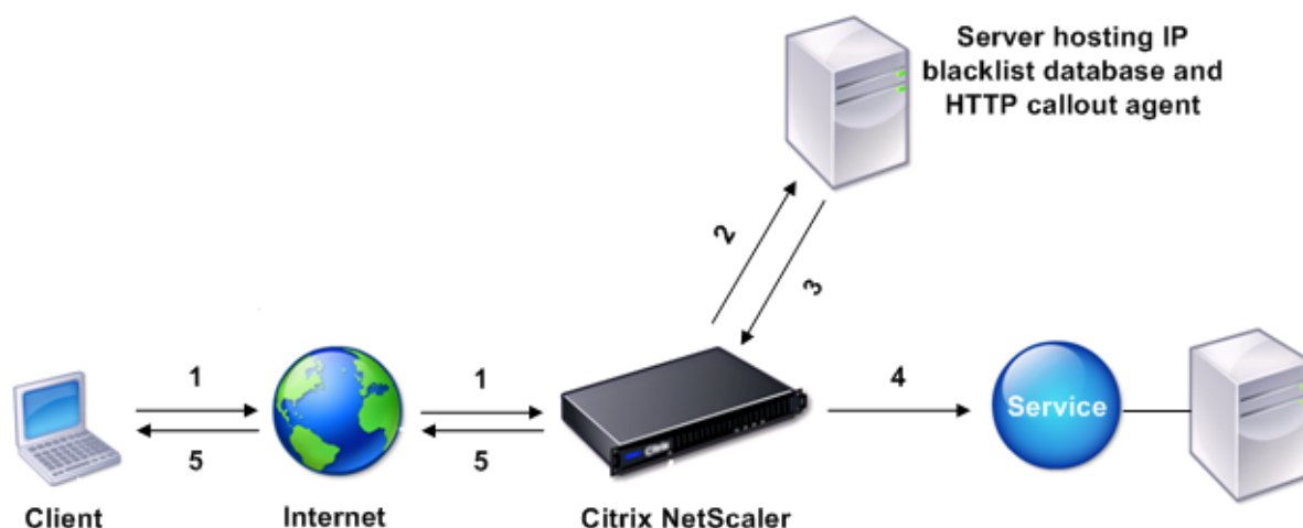
Abbildung 1. HTTP-Callout-Entitätsmodell
